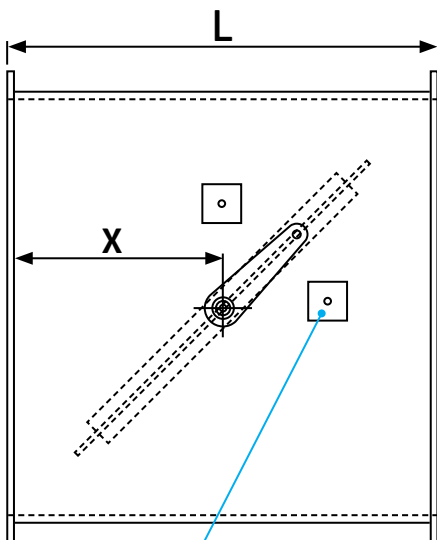
Arretierung auf/zu
