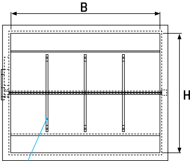
Verstärkungsrippen
