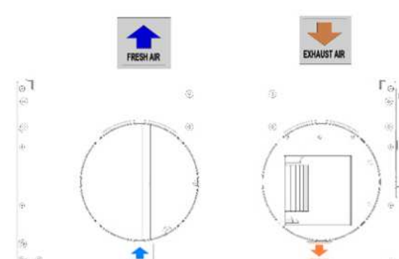
(Skizze zeigt zeigt AHU-300/400 HH)
