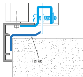
Klemme (KC)
