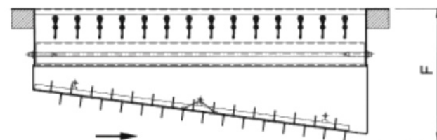
doppelreihiges Kanalgitter mit Schlitzschieber gerade
