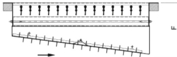
doppelreihiges Kanalgitter mit Schlitzschieber schräg
