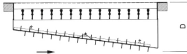
einreihiges Kanalgitter mit Schlitzschieber schräg
